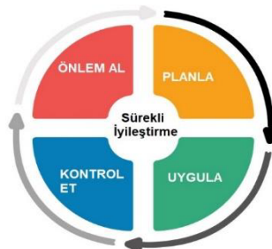
Şekil 1. PUKÖ Döngüsü
